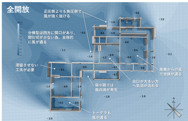
図3 石垣島を家のCFD解析
