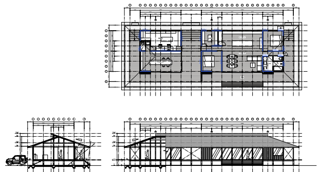
図4 計画図
