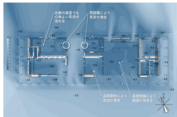
図6 設計提案のCFD解析
