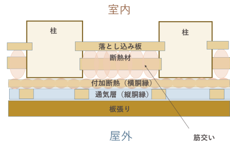
図3：壁の構成
