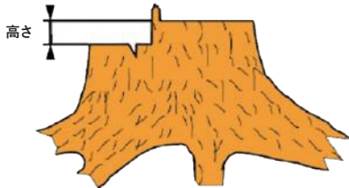
ツルの手前を切り下げ
