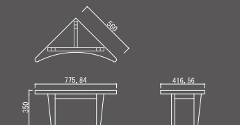
円八(嫁)図面 1/50
